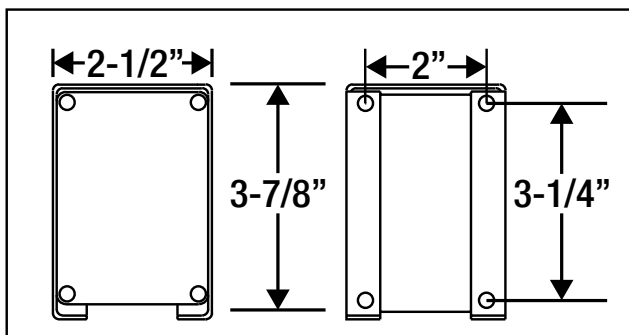
Photocell Module
